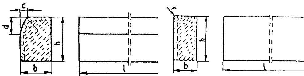
a) Krawężnik typu ulicznego
