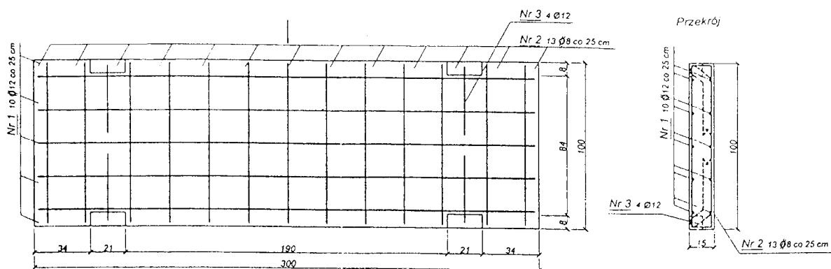
c) Płyta 3,0 \times 1,5 \times 0,18 m
