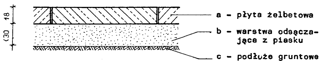
Rys. 5. Przykładowy przekrój poprzeczny nawierzchni z płyt
