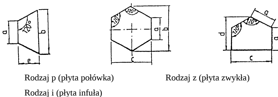
Rysunek 1. Kształt płyt betonowych
