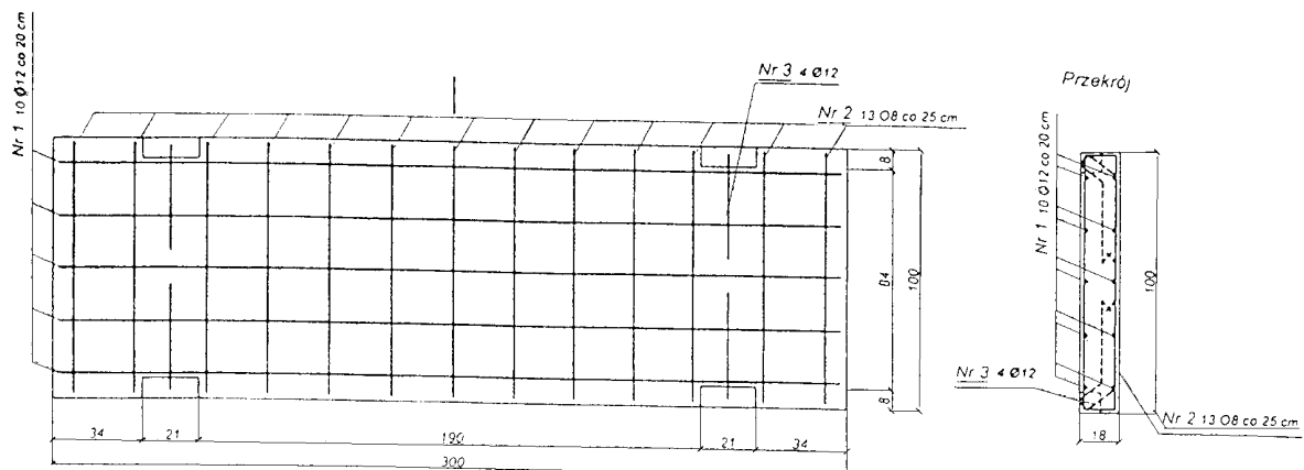
d) Płyta 3,0 \times 1,0 \times 0,18 m
