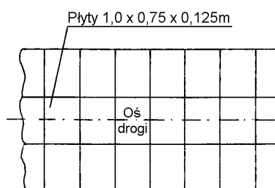
c) System płytowy nawierzchni szerokości 3 m – wariant 1 (płyty prostopadłe do osi drogi)
